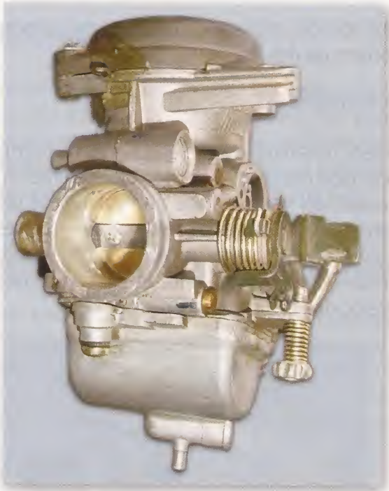
Carburador de mariposa y venturi invariable
